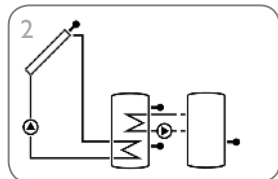
Zonnestelsysteem met warmtewisseling (pagina 11)
