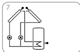
Zonnestelsysteem met 2 collectoren en 1 boiler (pagina 31)
