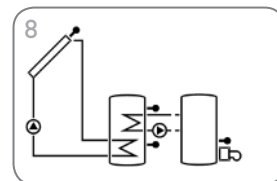
Zonnestelsysteem met naverwarming door vaste-brandstofketel (pagina 34)
