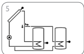
Zonnestelsysteem met 2 boilers met kleplogica (pagina 25)
