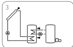
Zonnestelsysteem met naverwarming (pagina 17)
