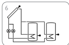
Zonnestelsysteem met 2 boilers met pomplogica (pagina 28)
