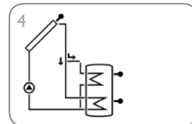
Zonnestelsysteem met gelaagde buffering (pagina 22)
